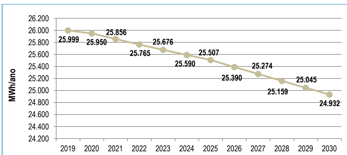
Figura 14. Consumos de energia no Município da Sertão: Setor dos Serviços (2019-2030)
