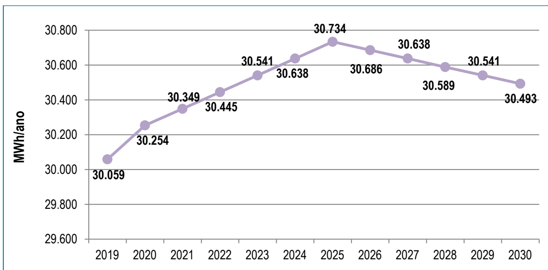
Figura 13. Consumos de energia no Município da Sertão: Setor Doméstico (2019-2030)
