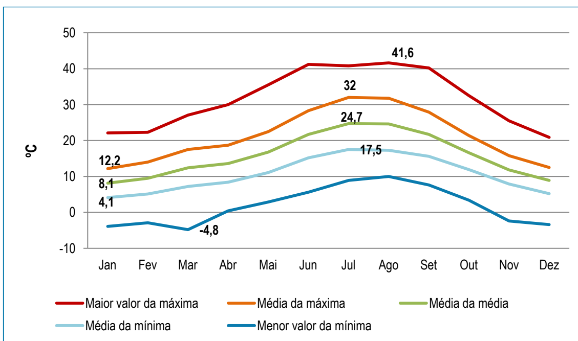
Figura 6. Temperatura do ar, normais climatológicas 1981-2010 (Castelo Branco)
