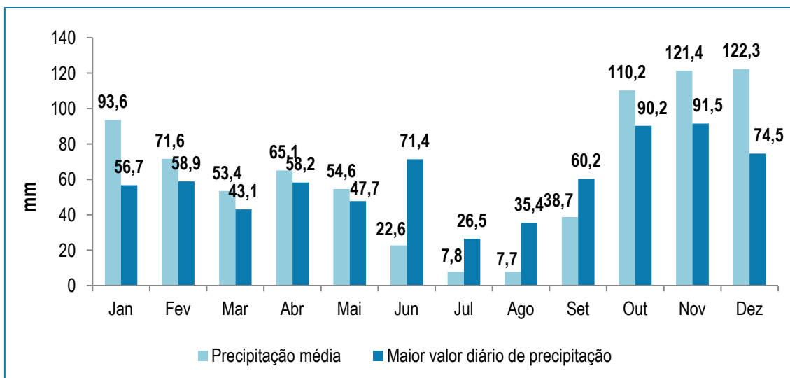
Figura 8. Precipitação, normais climatológicas 1981-2010 (Castelo Branco)
