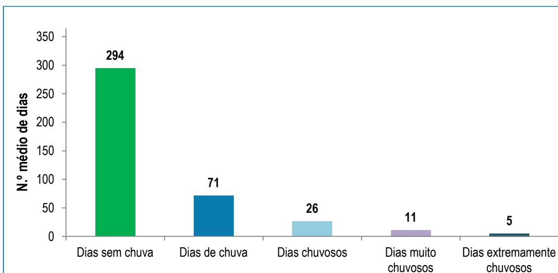
Figura 9. Precipitação (número médio de dias), normais climatológicas 1981-2010 (Castelo Branco)
