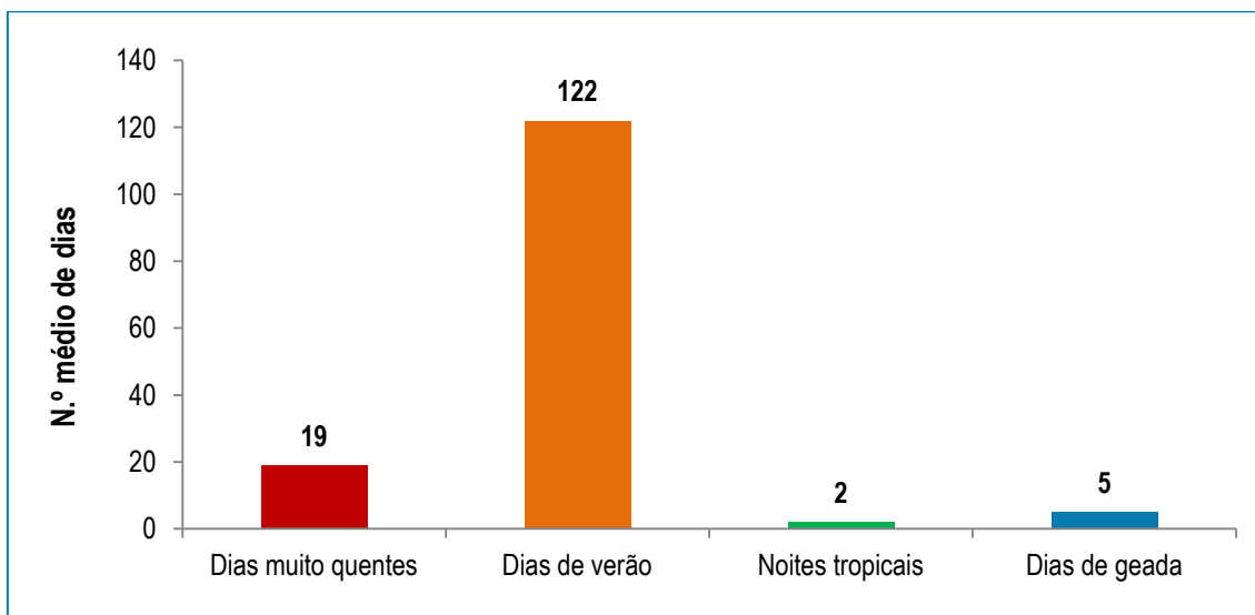
Figura 7. Temperatura do ar (número médio de dias), normais climatológicas 1981-2010 (Castelo Branco)
