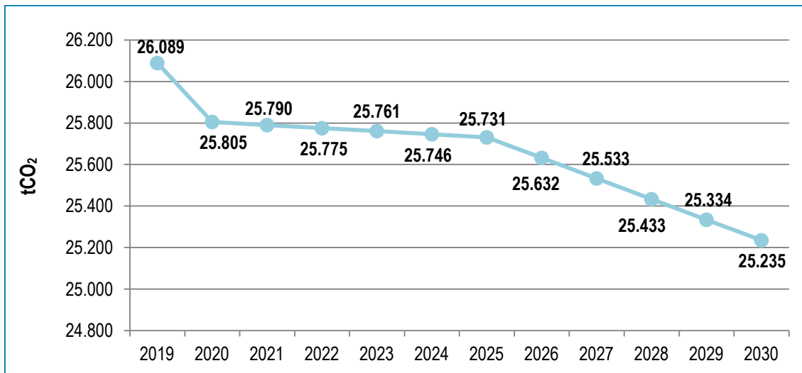
Figura 25. Emissões de GEE no Município da Sertão: Setor dos Transportes (2019-2030)
