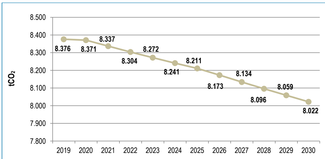
Figura 22. Emissões de GEE no Município da Sertão: Setor dos Serviços (2019-2030)
