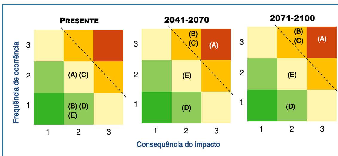
Figura 27. Evolução do risco climático do Município da Sertão
