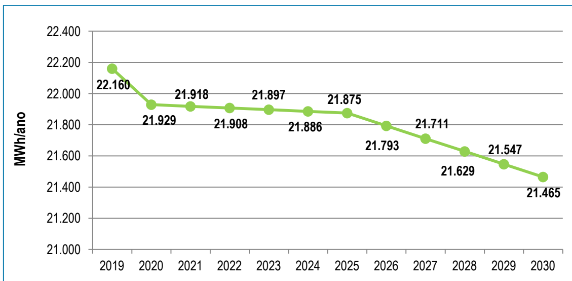
Figura 16. Consumos de energia no Município da Sertão: Setor da Agricultura (2019-2030)
