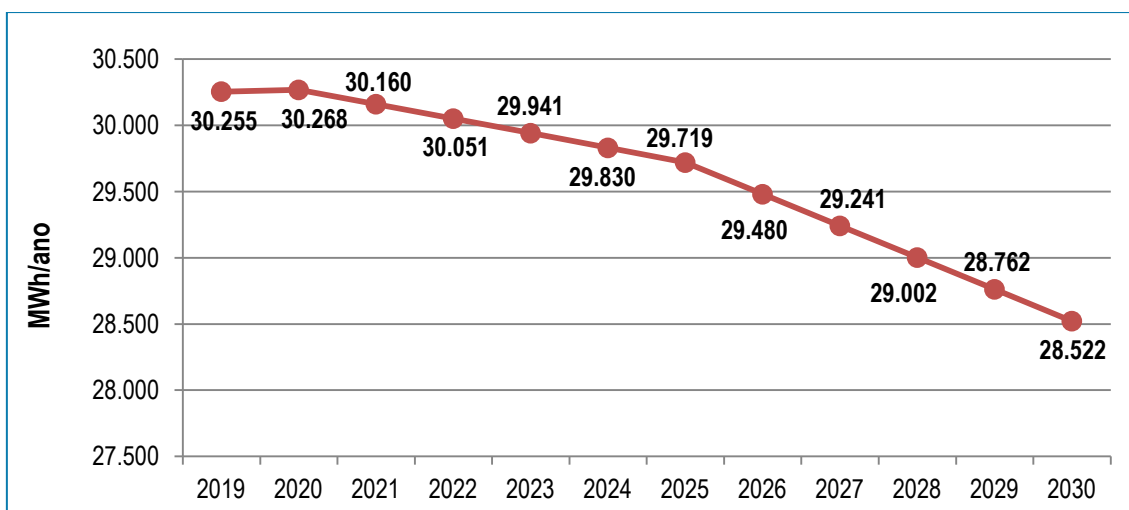
Figura 15. Consumos de energia no Município da Sertão: Setor da Indústria (2019-2030)
